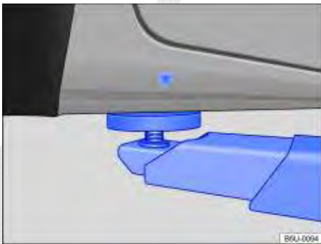
Fig. 122 Pontos de apoio dianteiros para a suspensão com plataforma elevatória ou com macaco.
