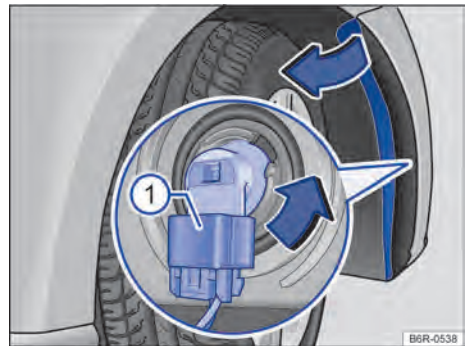
Fig. 146 Substituir a lâmpada incandescente do farol.
