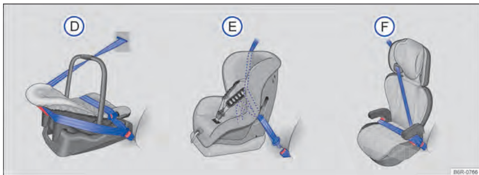
Fig. 49 As ilustrações (D), (E) e (F) mostram a fixação do sistema de retenção para crianças apenas com o cinto de segurança do veículo.
