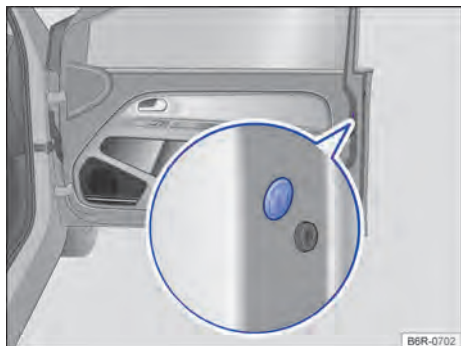
Fig. 130 Na parte dianteira da porta do passageiro dianteiro: travamento de emergência, coberto por uma vedação de borracha.
