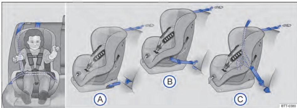
Fig. 48 No banco traseiro: as figuras A e B mostram o princípio da fixação do sistema de retenção para crianças nos olhais de retenção inferiores e com o cinto de fixação superior. A figura C mostra a fixação do sistema de retenção para crianças com o cinto de segurança do veículo e com o cinto de fixação superior.
