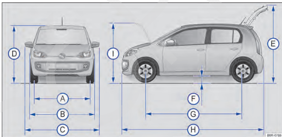
Fig. 158 Dimensões.
