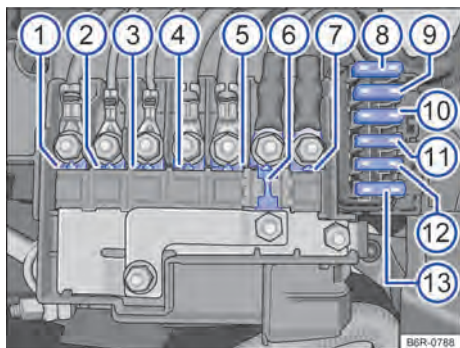
Fig. 145 Caixa de fusíveis.
