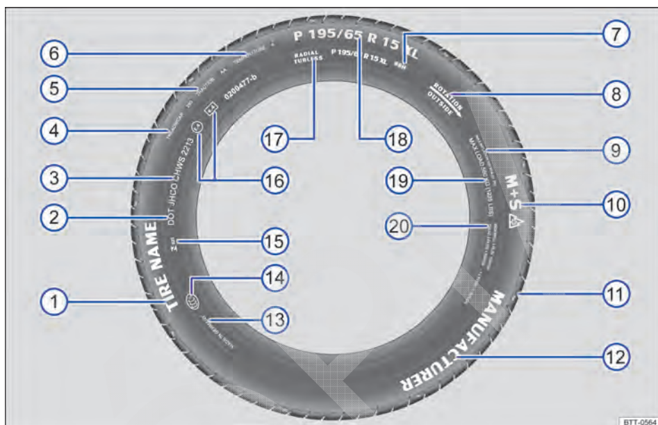
Fig. 119 Inscrição dos pneus internacional (exemplo).
