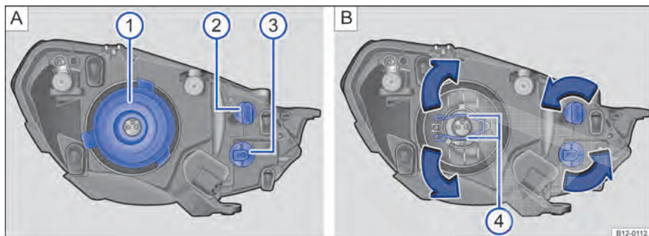
Fig. 146 No compartimento do motor: vista traseira do farol dianteiro esquerdo com cobertura de borracha: ① farol baixo e farol alto, ② luz de posição, ③ indicadores de direção e trava de proteção ④.
