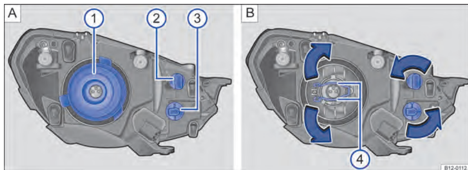
Fig. 110 No compartimento do motor: vista traseira do farol dianteiro esquerdo com cobertura de borracha: ① farol baixo e farol alto, ② luz de posição e/ou luz de condução diurna, ③ indicadores de direção e trava de proteção ④.
