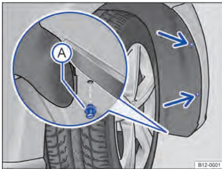
Fig. 111 Na caixa da roda dianteira direita: remover os parafusos de fixação (setas) e remover o rebite de expansão (A).
