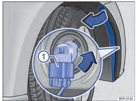
Fig. 112 Substituir a lâmpada incandescente do farol.
