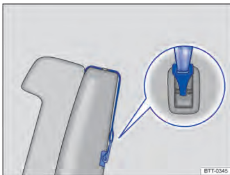
Fig. 36 Exemplo de um cinto de fixação superior preso.
