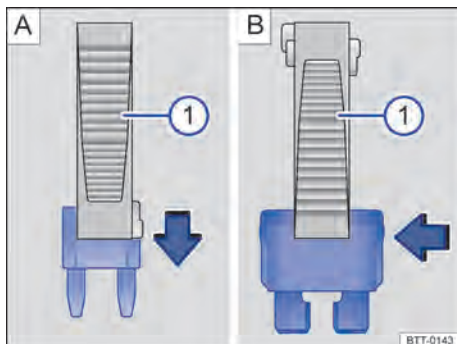
Fig. 122 Remover ou instalar um fusível com a garra da pinça de plástico ①.
