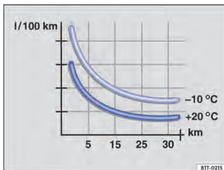
Fig. 78 Consumo de combustível em l/100 km em 2 temperaturas ambiente diferentes.
