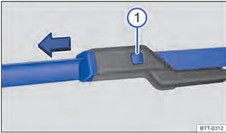
Fig. 127 Substituir as palhetas dos limpadores do para-brisa.
