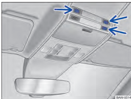
Fig. 57 No console do teto: sensores de monitoramento do interior do veículo (setas).
