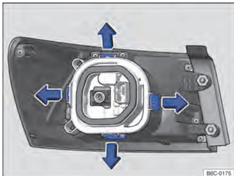
Fig. 134 Lanterna traseira: desinstalar o suporte das lâmpadas
