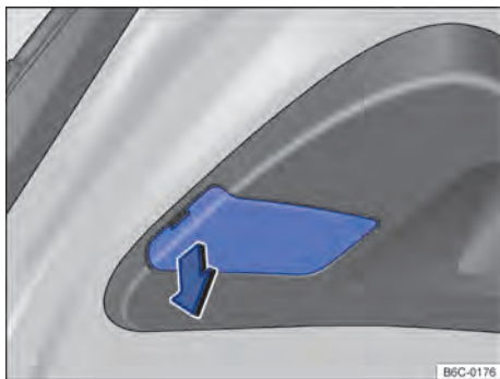
Fig. 135 Na tampa traseira: desmontar a cobertura da lanterna traseira.
