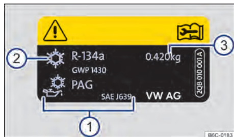
Fig. 175 Informações do ar-condicionado - motor 1.0L TSI e motor 1.6L.
