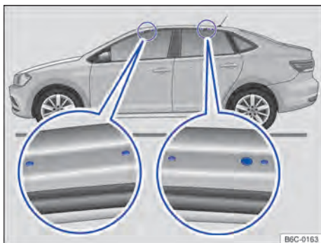
Fig. 120 Pontos de fixação dos suportes de base do bagageiro do teto (ambos os lados).
