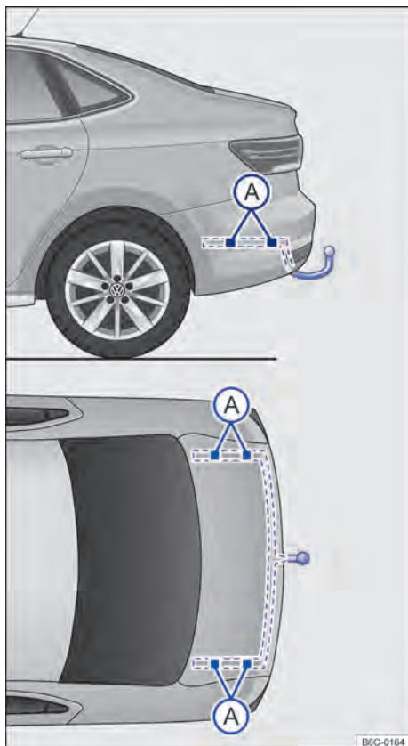
Fig. 121 Pontos de fixação para instalar um dispositivo de reboque posteriormente.
