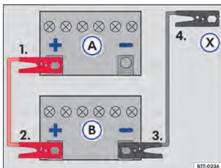
Fig. 146 Esquema para a conexão dos cabos auxiliares de partida: bateria do veículo descarregada (A) e bateria do veículo fornecedora de corrente (B).
