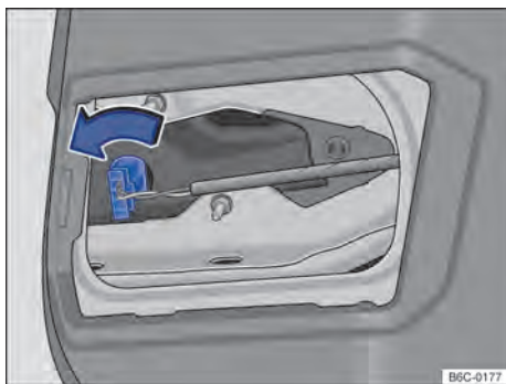
Fig. 136 Na tampa traseira: desinstalar o suporte da lâmpada.
