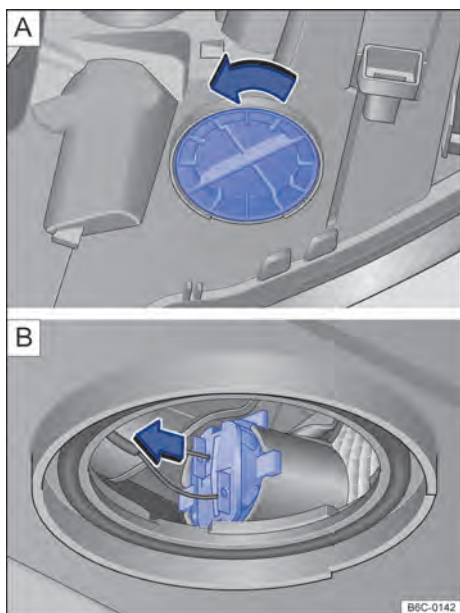
Fig. 130 Farol dianteiro, por baixo: cobertura do indicador de direção.
