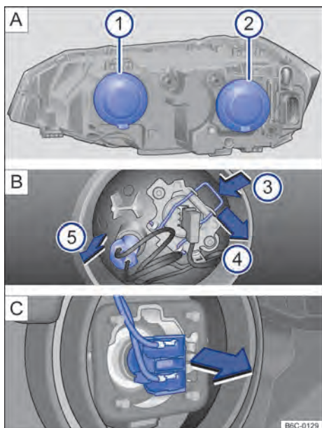
Fig. 129 No compartimento do motor: ① farol alto e luz de posição e ② farol baixo.
