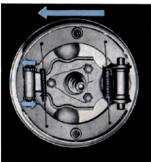
Roda dianteira
