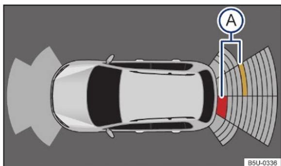
Fig. 92 Exibição do display do controle de distância de estacionamento traseiro no aparelho de navegação (não disponível para algumas versões).
