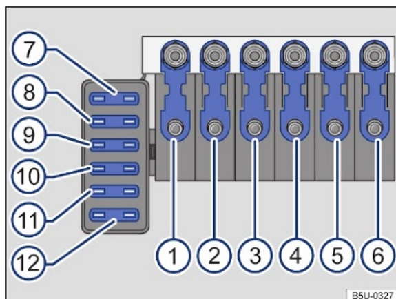
Fig. 120 Caixa de fusíveis.
