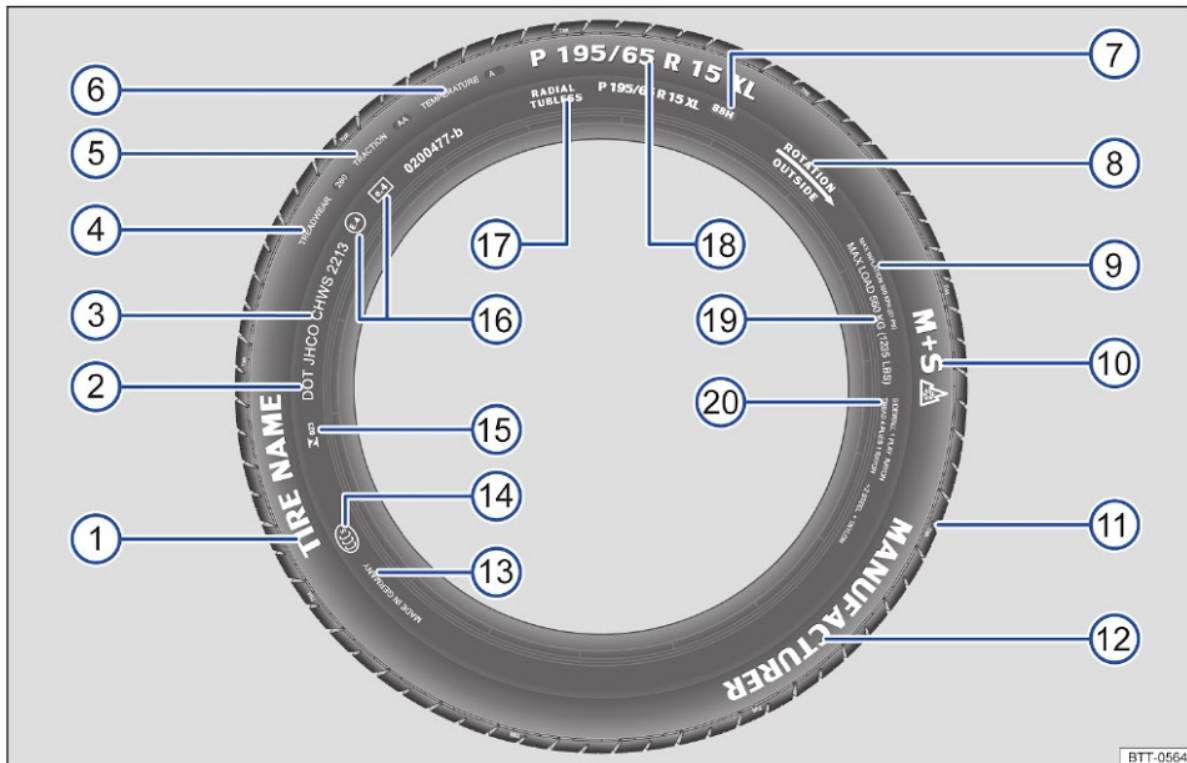
Fig. 140 Inscrição dos pneus internacional (exemplo).
