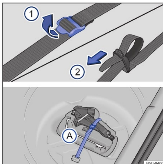
Fig. 104 No compartimento de bagagem: cinta de fixação da caixa de ferramentas e caixa de ferramentas de bordo.
