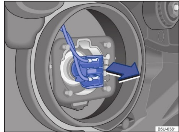
Fig. 111 Acesso à lâmpada incandescente do farol baixo.
