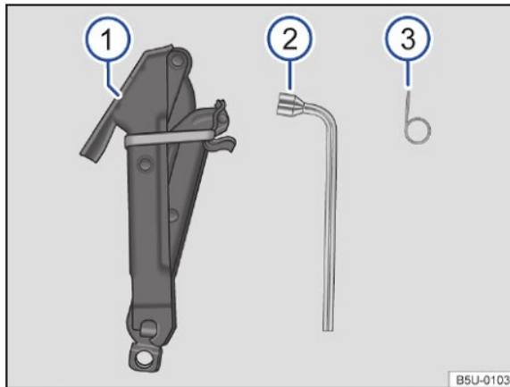
Fig. 105 Componentes das ferramentas de bordo.
