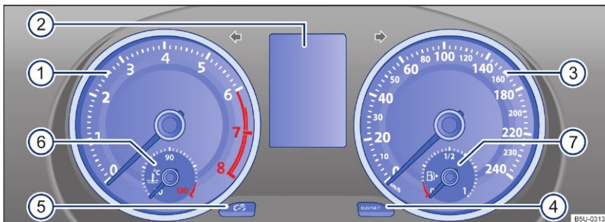
Fig. 12 Instrumento combinado no painel de instrumentos (variante 2).
