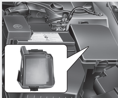
Painel de fusíveis do compartimento do motor
