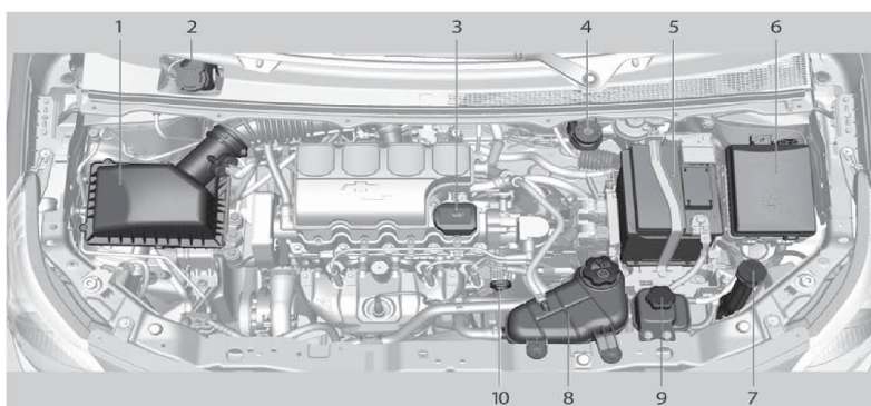
Motor ECONO.FLEX
