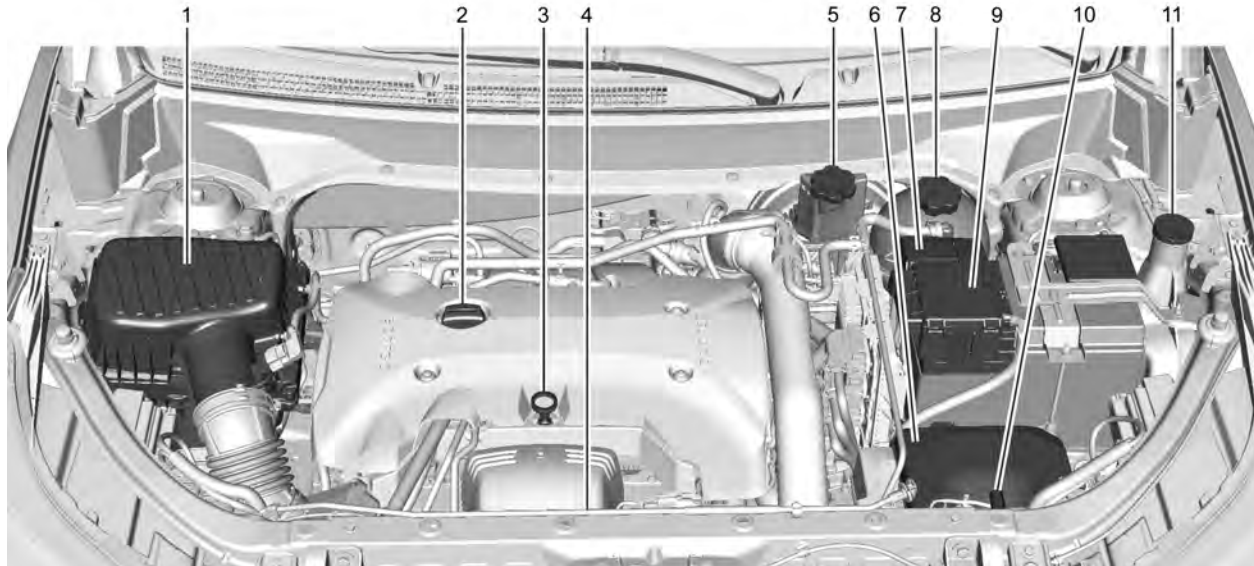
Motor 2.0L
