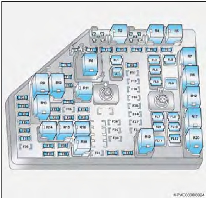
Caixa de fusíveis e relés do compartimento do motor – capacidades (ampère) e circuitos elétricos protegidos
