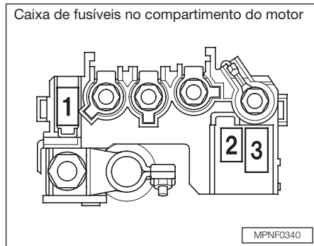
Caixa de fusíveis no compartimento do motor
