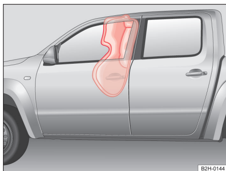
Fig. 39 Área de expansão do airbag para cabeça e laterais combinado no lado esquerdo do veículo.
