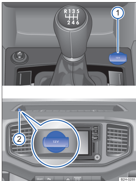
Fig. 124 Tomada 12 V: no console central dianteiro 1 e no porta-objetos no painel de instrumentos 2.
