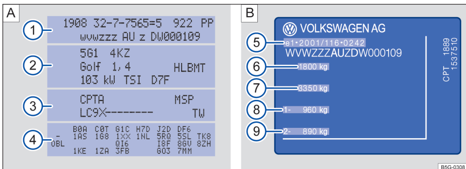
Fig. 206 A) Etiqueta de dados do veículo: na figura de exemplo com o código do motor CPTA ③. B) Plaqueta de identificação.
