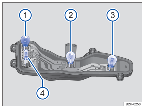
Fig. 152 Suporte da lâmpada: 1 indicadores de direção, 2, lanterna traseira, 3 lanterna de freio, 4 Dependendo da versão, lanterna de marcha a ré ou suporte da lâmpada à direita lanterna de marcha a ré e suporte da lâmpada à esquerda lanterna de neblina.
