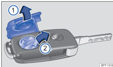
Fig. 47 Chave do veículo: substituir a pilha botão.
