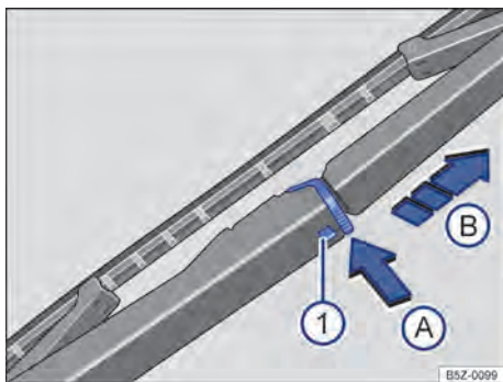
Fig. 148 Substituir a palheta do limpador do vidro traseiro.
