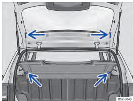
Fig. 138 No compartimento de bagagem: remover e instalar a cobertura do compartimento de bagagem.
