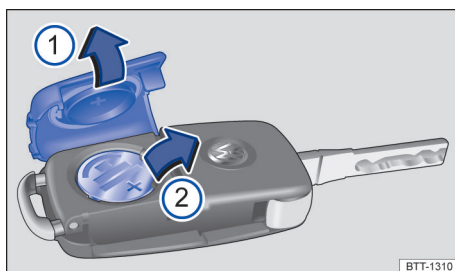
Fig. 54 Chave do veículo com comando remoto: 1) Abrir a tampa do alojamento da bateria. 2) Remover a bateria.
