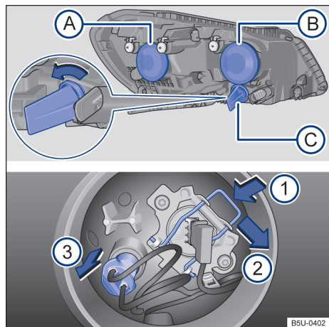
Fig. 159 No compartimento do motor: vista traseira do farol dianteiro com cobertura de borracha (lado esquerdo da ilustração) - A farol baixo, B farol alto e luz de posição, e C indicador de direção. Vista traseira do farol dianteiro sem a cobertura de borracha (lado direito da ilustração): 1 mola de travamento da lâmpada incandescente do farol e 2 luz de posição.
