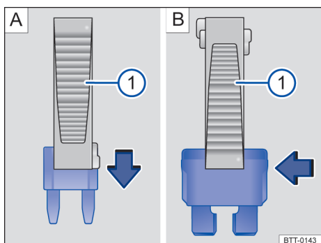
Fig. 175 Remover ou instalar um fusível com a garra da pinça de plástico ⓘ.
