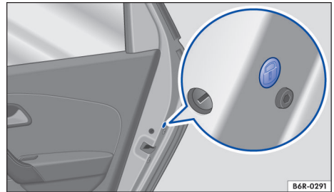
Fig. 60 Na parte dianteira da porta direita: travamento de emergência, coberto por uma vedação de borracha.
