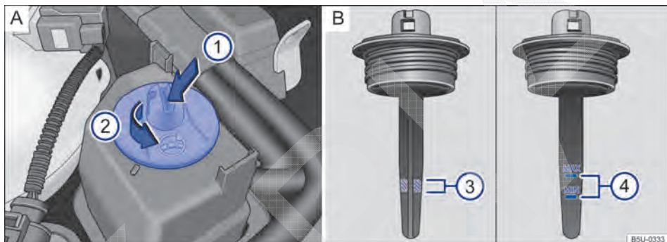
Fig. 108 No compartimento do motor (variante 1): A Reservatório do fluido da direção hidráulica. B Marcações para controle do nível do fluido da direção hidráulica.
