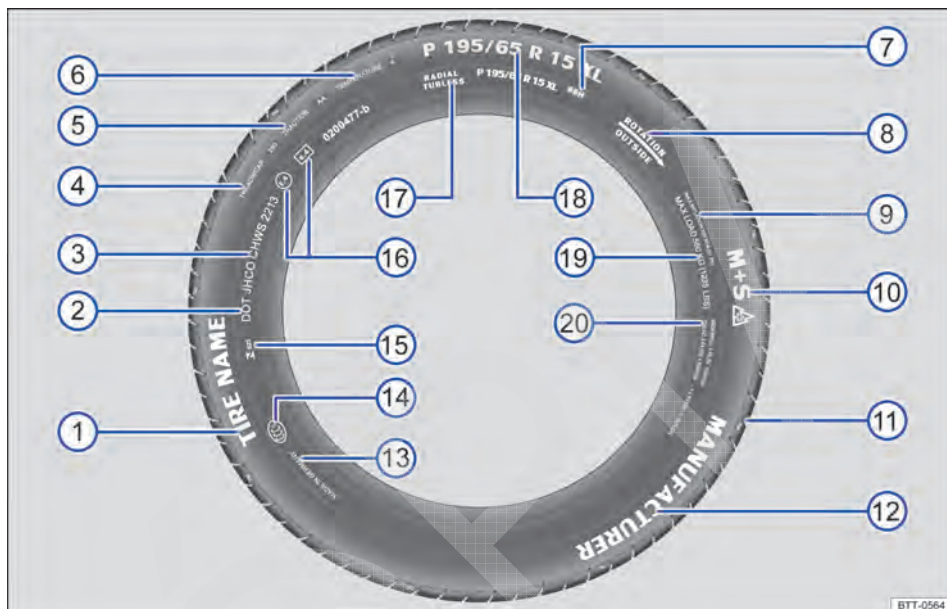
Fig. 137 Inscrição dos pneus internacional (exemplo).
