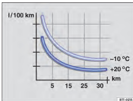
Fig. 107 Consumo de combustível em l/100 km em 2 temperaturas ambiente diferentes.
