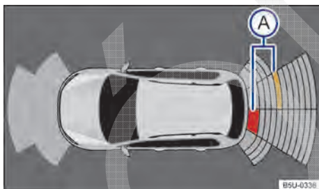
Fig. 112 Exibição do display do controle de distância de estacionamento traseiro no aparelho de navegação (não disponível para algumas versões).
