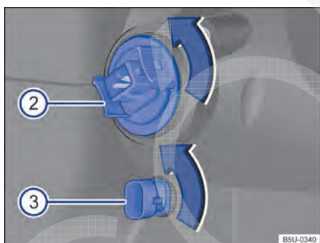
Fig. 169 No compartimento do motor: vista traseira do farol dianteiro (2) indicadores de direção e (3) luz de posição.
