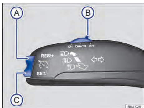
Fig. 114 À esquerda na coluna da direção: alavanca de operação do GRA.
