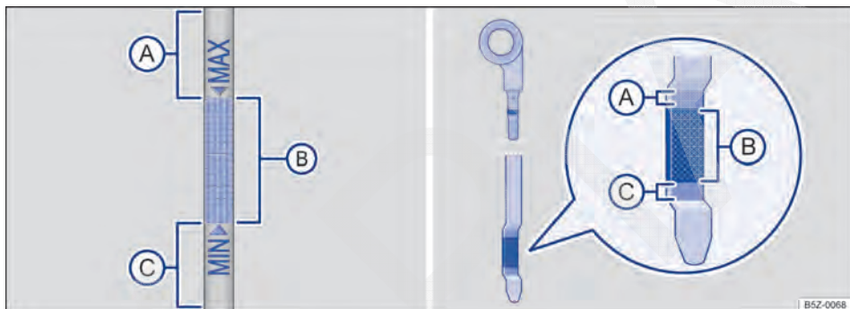
Fig. 124 Vareta de medição do óleo com marcas de nível do óleo do motor.
