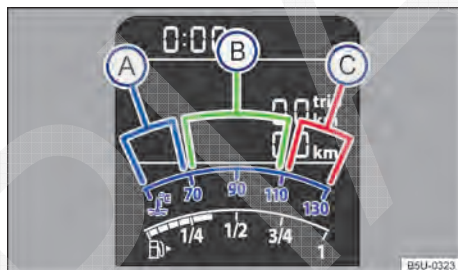
Fig. 126 Indicador de temperatura do líquido de arrefecimento do motor no instrumento combinado (variante 1): (A) área fria; (B) área normal; (C) área de alerta.
