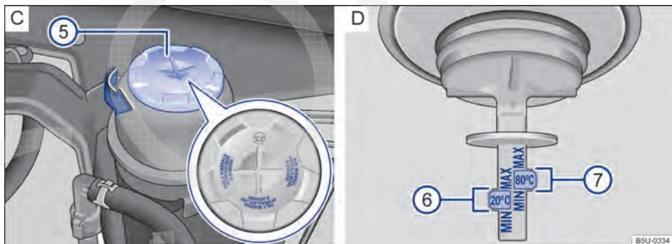
Fig. 109 No compartimento do motor (variante 2): C Reservatório do fluido da direção hidráulica. D Marcações para controle do nível do fluido da direção hidráulica.
