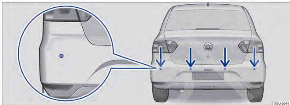
Fig. 110 Sensores de ultrassom do controle de distância de estacionamento no para-choque traseiro.
