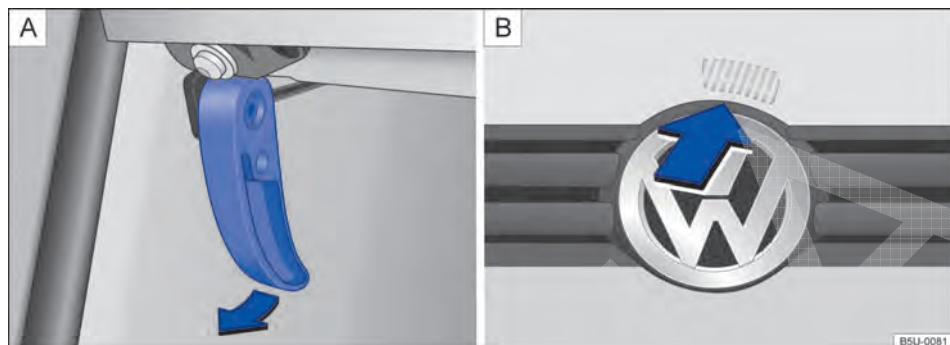
Fig. 122 A Alavanca de destravamento da tampa do compartimento do motor na área para os pés do lado do condutor. B Alavanca de destravamento na parte interna da tampa do compartimento do motor.
