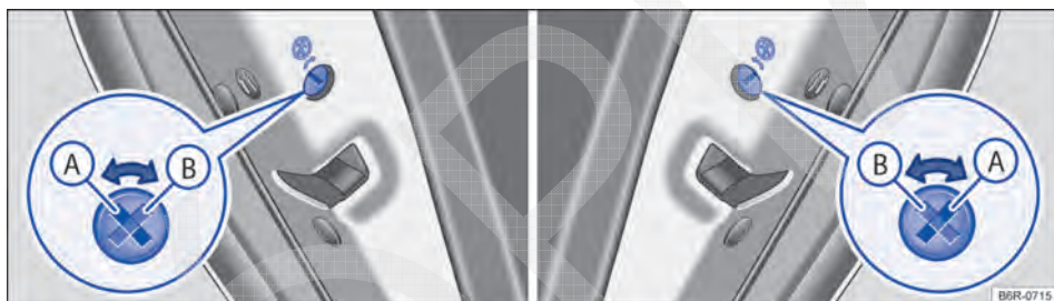
Fig. 57 Nas portas traseiras: trava de segurança para crianças (A) desacionada, (B) acionada.
