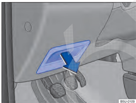
Fig. 162 No lado do condutor no painel de instrumentos: cobertura da caixa de fusíveis.
