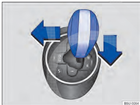
Fig. 100 Alavanca seletora da transmissão automatizada ASG.
