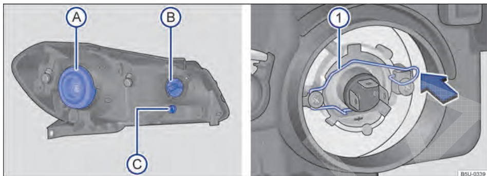
Fig. 168 No compartimento do motor: vista traseira do farol dianteiro com cobertura de borracha (lado esquerdo da ilustração) - (A) farol baixo / alto, (B) indicadores de direção e (C) luz de posição. Vista traseira do farol dianteiro sem a cobertura de borracha (lado direito da ilustração): (1) mola de travamento da lâmpada incandescente do farol baixo / alto.
