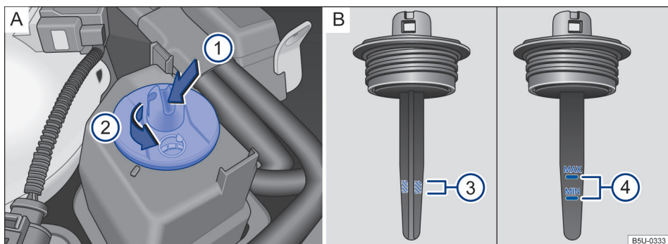
Fig. 89 No compartimento do motor (variante 1): A Reservatório do fluido da direção hidráulica. B Marcações para controle do nível do fluido da direção hidráulica.
