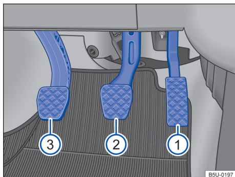
Fig. 77 Na área para os pés: pedais em veículos com transmissão manual.
