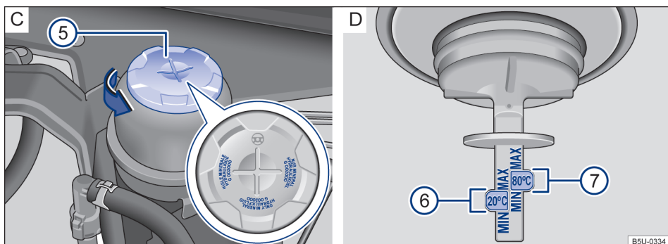
Fig. 90 No compartimento do motor (variante 2): C Reservatório do fluido da direção hidráulica. D Marcações para controle do nível do fluido da direção hidráulica.
