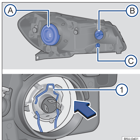
Fig. 109 No compartimento do motor: vista traseira do farol dianteiro com cobertura de borracha (lado esquerdo da ilustração) - (A) farol baixo / alto, (B) indicadores de direção e (C) luz de posição. Vista traseira do farol dianteiro sem a cobertura de borracha (lado direito da ilustração): (1) mola de travamento da lâmpada incandescente do farol baixo / alto.
