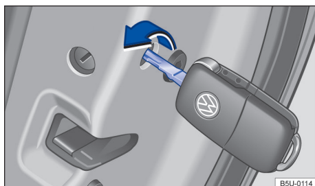
Fig. 52 Travamento de emergência do veículo com a chave do veículo.
