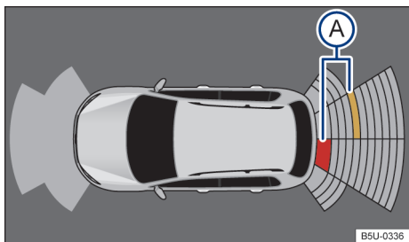
Fig. 93 Exibição do display do controle de distância de estacionamento traseiro no aparelho de navegação (não disponível para algumas versões).
