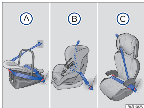
Fig. 37 As ilustrações (A), (B) e (C) mostram a fixação do sistema de retenção para crianças apenas com o cinto de segurança do veículo.
