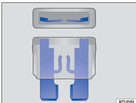
Fig. 123 Representação de um fusível queimado.
