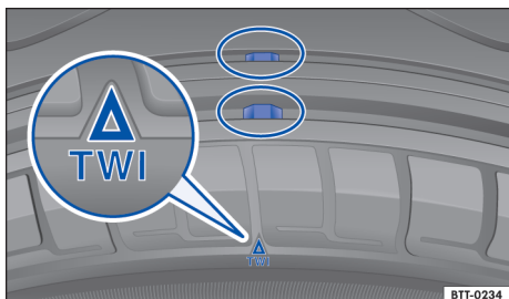
Fig. 140 Perfil do pneu: indicadores de desgaste.
