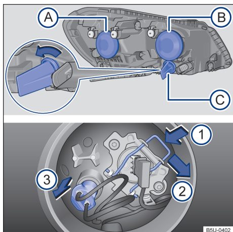
Fig. 111 No compartimento do motor: vista traseira do farol dianteiro com cobertura de borracha (lado esquerdo da ilustração) - (A) farol baixo, (B) farol alto e luz de posição, e (C) indicador de direção. Vista traseira do farol dianteiro sem a cobertura de borracha (lado direito da ilustração): ① mola de travamento da lâmpada incandescente do farol e ② luz de posição.
