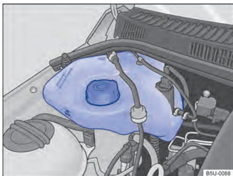
Fig. 180 No compartimento do motor: reservatório de gasolina para o sistema de partida a frio.
