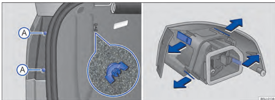
Fig. 161 Na carroceria: remover a lanterna traseira e suporte das lâmpadas.
