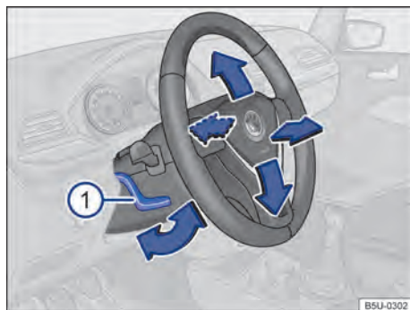
Fig. 53 Embaixo e à esquerda do volante junto com o revestimento da coluna de direção: alavanca de ajuste da posição do volante.
