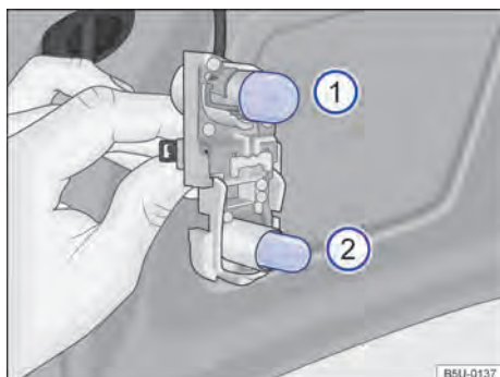
Fig. 160 No suporte das lâmpadas: localização das lâmpadas.
