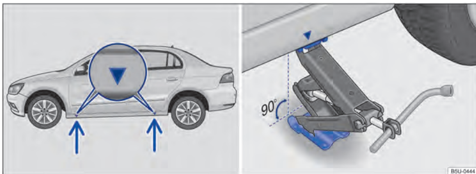
Fig. 191 Pontos de apoio do macaco e macaco posicionado no lado esquerdo traseiro do veículo.
