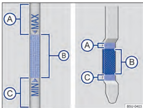
Fig. 175 Vareta de medição do óleo com marcas de nível do óleo do motor.
