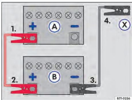
Fig. 171 Esquema para a conexão dos cabos auxiliares de partida: bateria do veículo descarregada (A) e bateria do veículo fornecedora de corrente (B).
