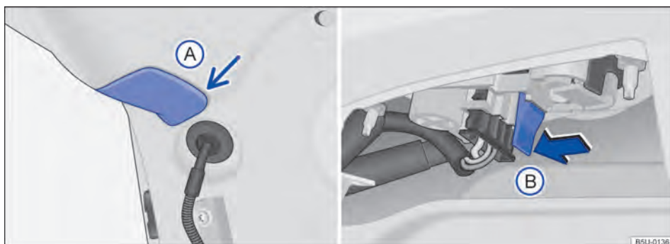
Fig. 159 Na tampa traseira: remover a cobertura e suporte das lâmpadas.
