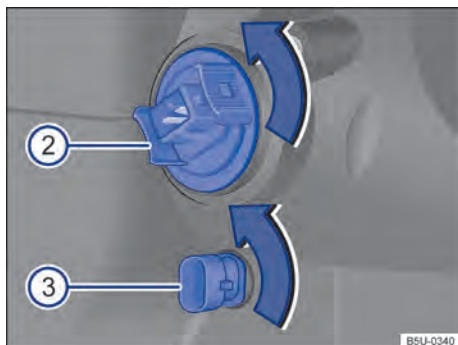
Fig. 155 No compartimento do motor: vista traseira do farol dianteiro (2) indicadores de direção e (3) luz de posição.
