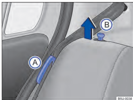
Fig. 56 Banco traseiro: posicionador do cadarço do cinto de segurança A e pino de destravamento do encosto B.
