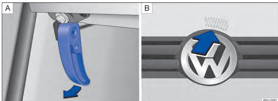
Fig. 172 A) Alavanca de destravamento da tampa do compartimento do motor na área para os pés do lado do condutor. B) Alavanca de destravamento na parte interna da tampa do compartimento do motor.
