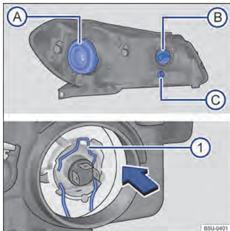
Fig. 154 No compartimento do motor: vista traseira do farol dianteiro com cobertura de borracha (lado esquerdo da ilustração) - (A) farol baixo / alto, (B) indicadores de direção e (C) luz de posição. Vista traseira do farol dianteiro sem a cobertura de borracha (lado direito da ilustração): (1) mola de travamento da lâmpada incandescente do farol baixo / alto.
