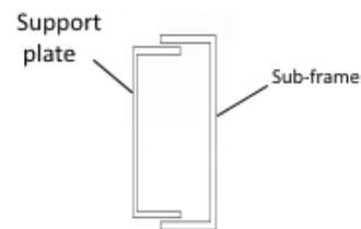
Exemplo utilizando uma placa de suporte
