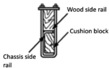
Exemplo com um bloco de madeira de suporte
