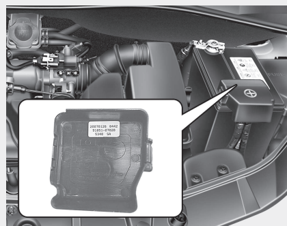
Painel secundário de fusíveis do compartimento do motor (Só veículos gasolina, se instalado)
