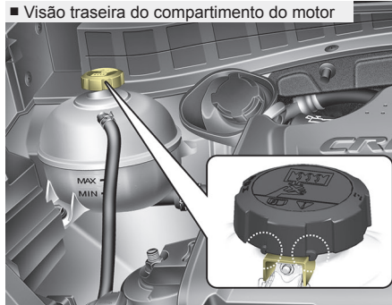
■ Visão traseira do compartimento do motor
